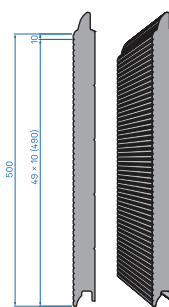
V-profil
